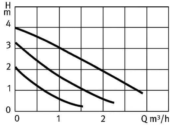
Kennlinien für NEHS® Umwälzpumpen N 25/70, N 32/70
