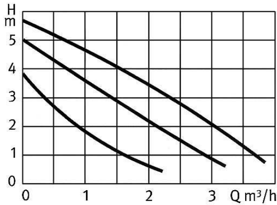
Kennlinien für NEHS® Umwälzpumpen NE-Plus 25/40, NE-Plus 32/40
