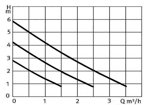
Kennlinien für NEHS® Umwälzpumpen NE-Plus 25/60, NE-Plus 32/60
