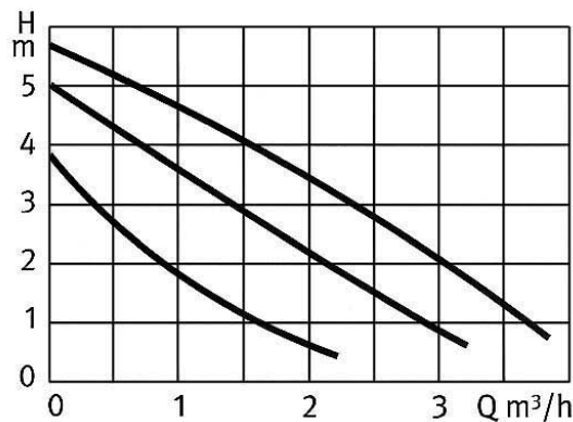
Kennlinien für NEHS® Solarpumpe SN 15/60
